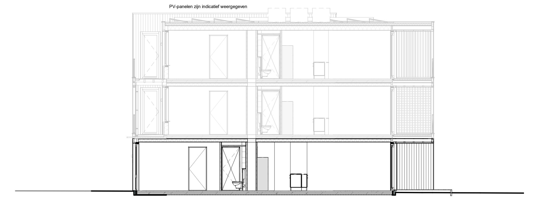
A-A - Zandheugel 23-24
