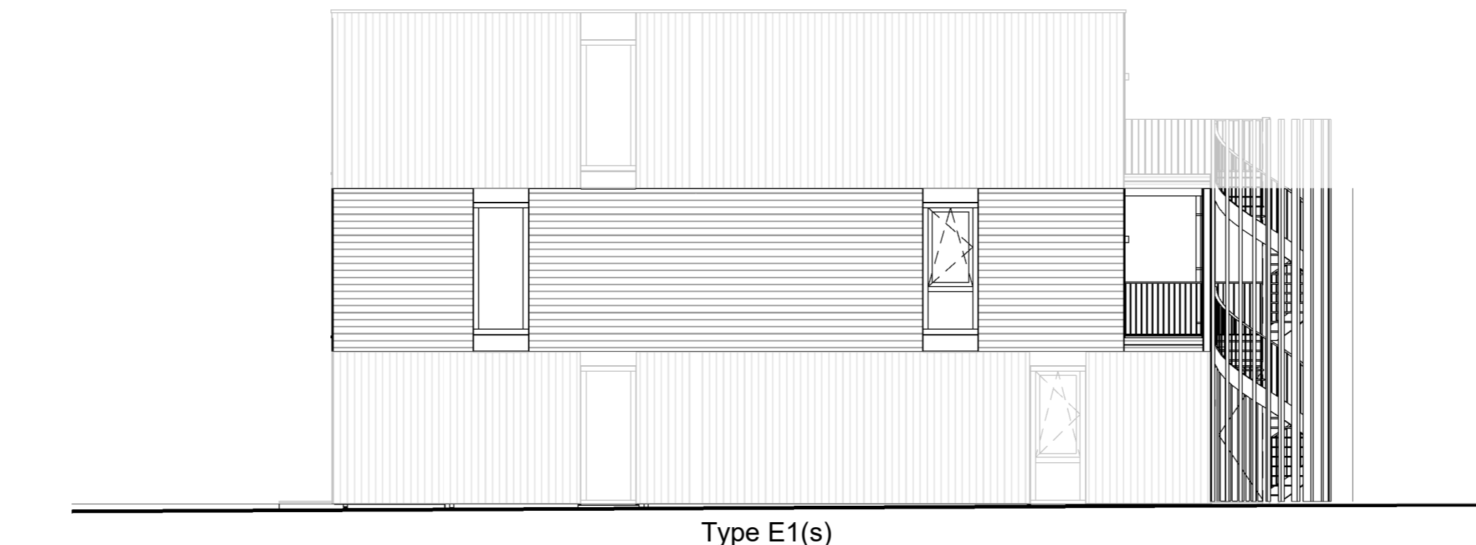
linker kopgevel - Zandheugel 36 Type E1(s) bwnr. Z36
