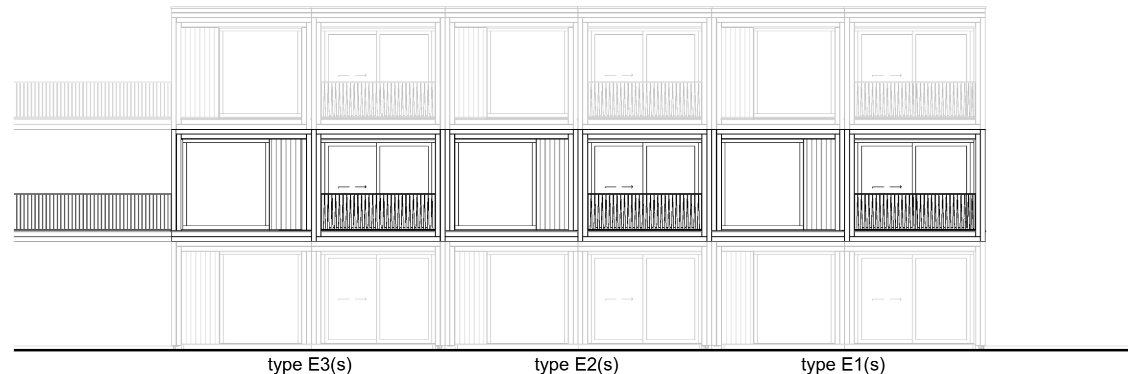
achtergevel - Zandheugel 34-36 type E3(s) bwnr. Z34 type E2(s) bwnr. Z35 type E1(s) bwnr. Z36
